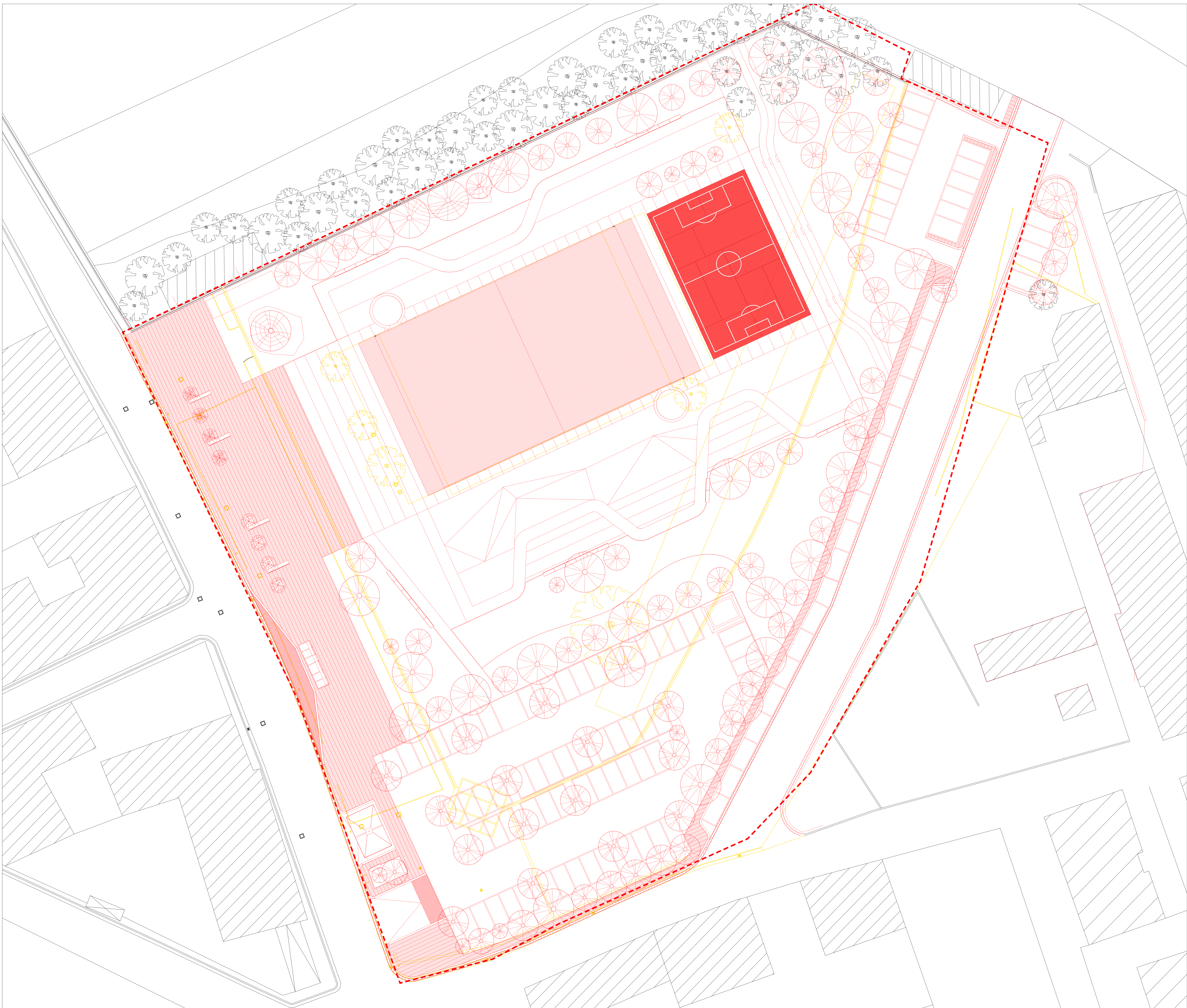
Pianta demolizioni e ricostruzioni - scala 1:200
